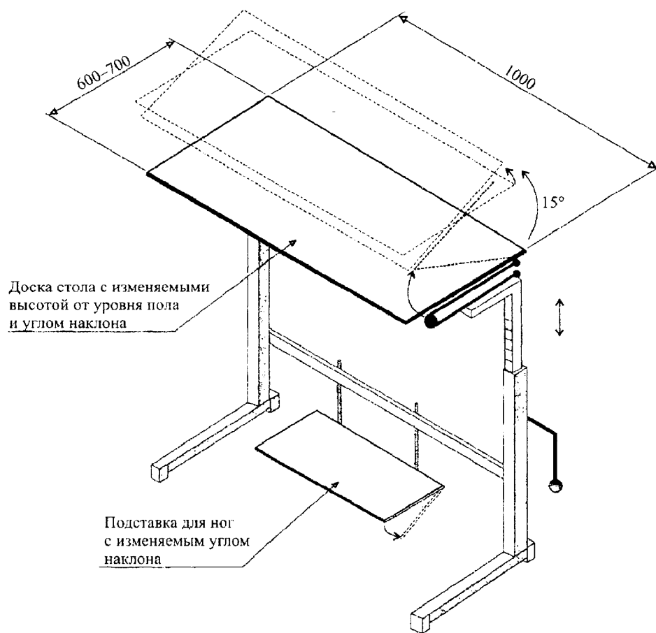
Рисунок В.12. Трансформируемый рабочий стол для инвалида
