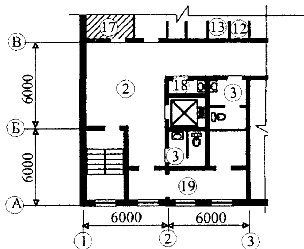
Фрагмент плана на отм. 4.800
