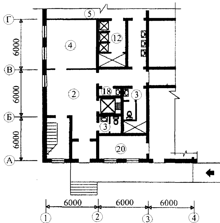
Фрагмент плана на отм. 4.800
