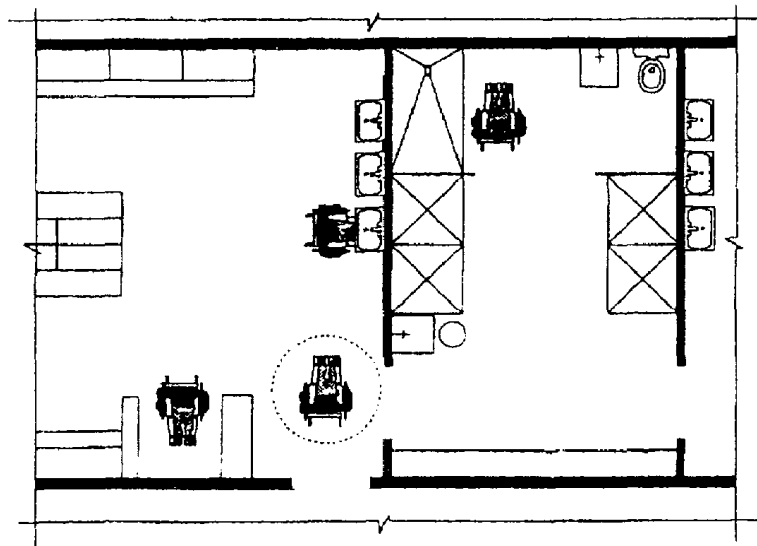
Размещение гардеробной (а) и душевой (б) для инвалидов в общем гардеробном блоке. Индивидуальная кабина инвалида в общей душевой
