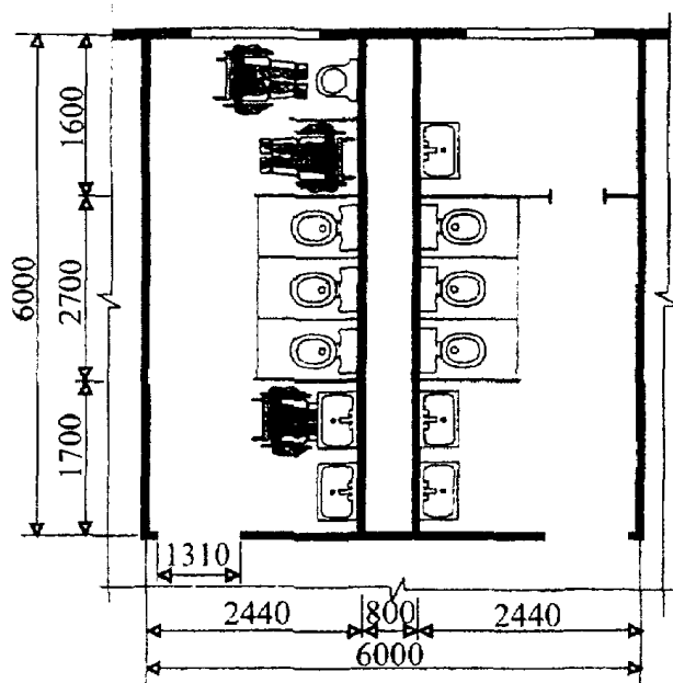
Цеховая уборная с кабиной для инвалидов
