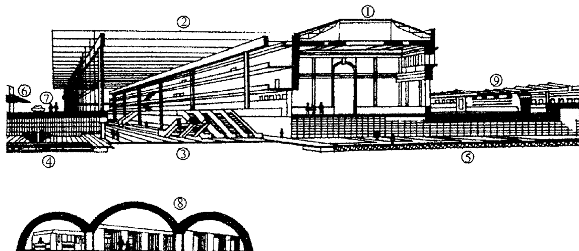
Поперечный разрез по зданию вокзала, перрону и привокзальной площади
